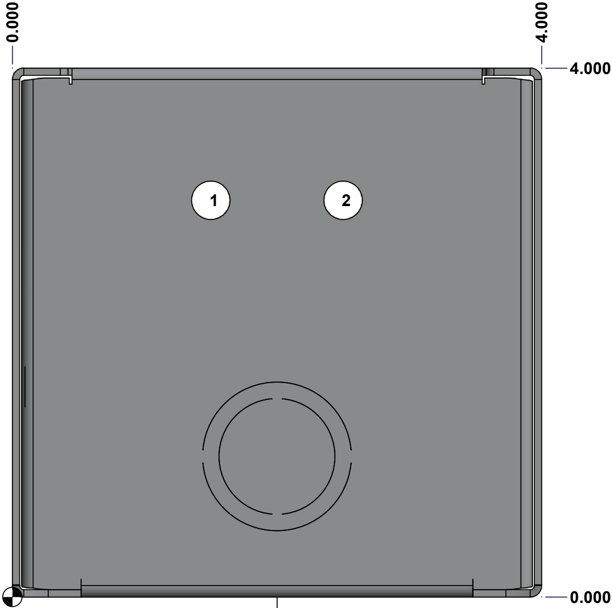
BOTTOM
