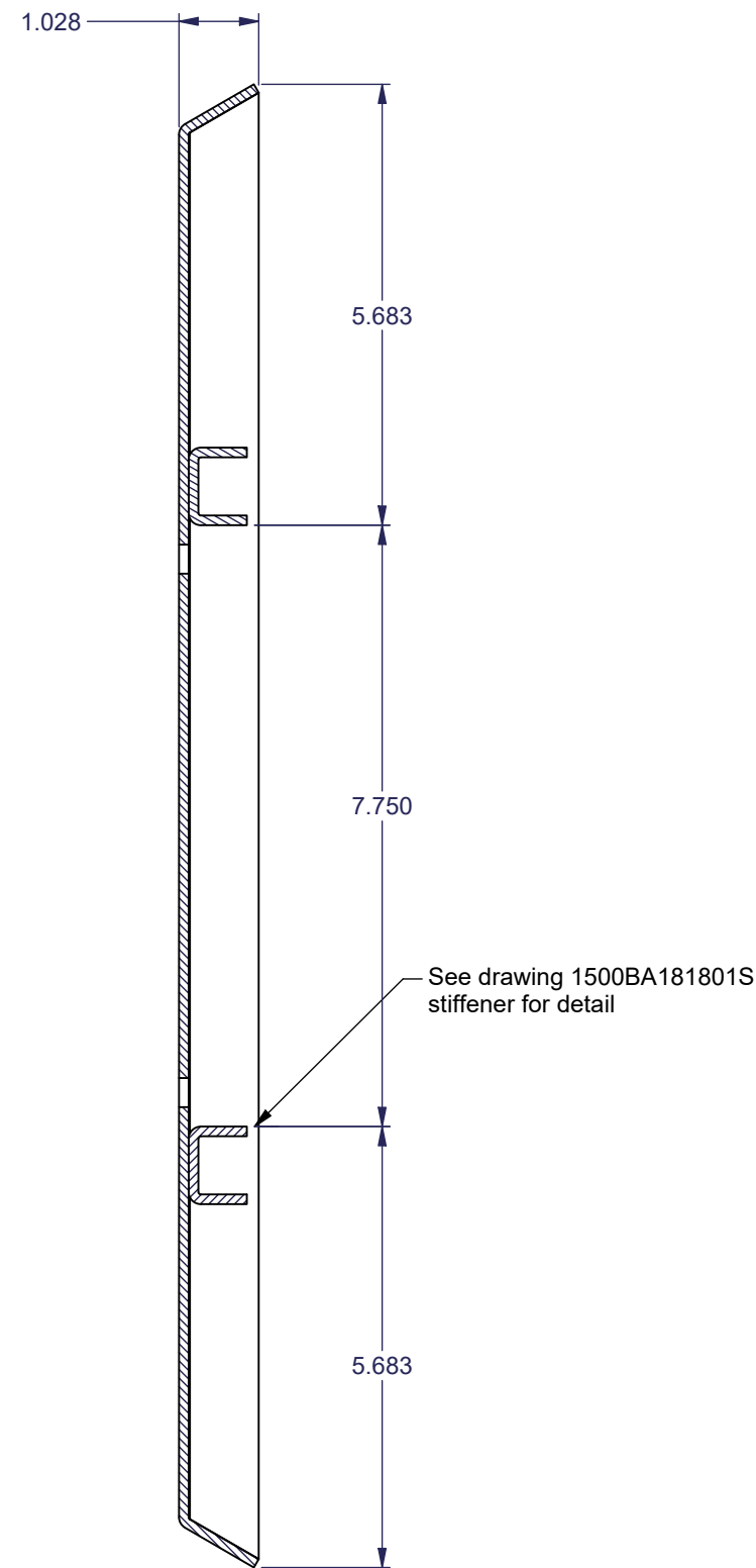
SECTION A-A
