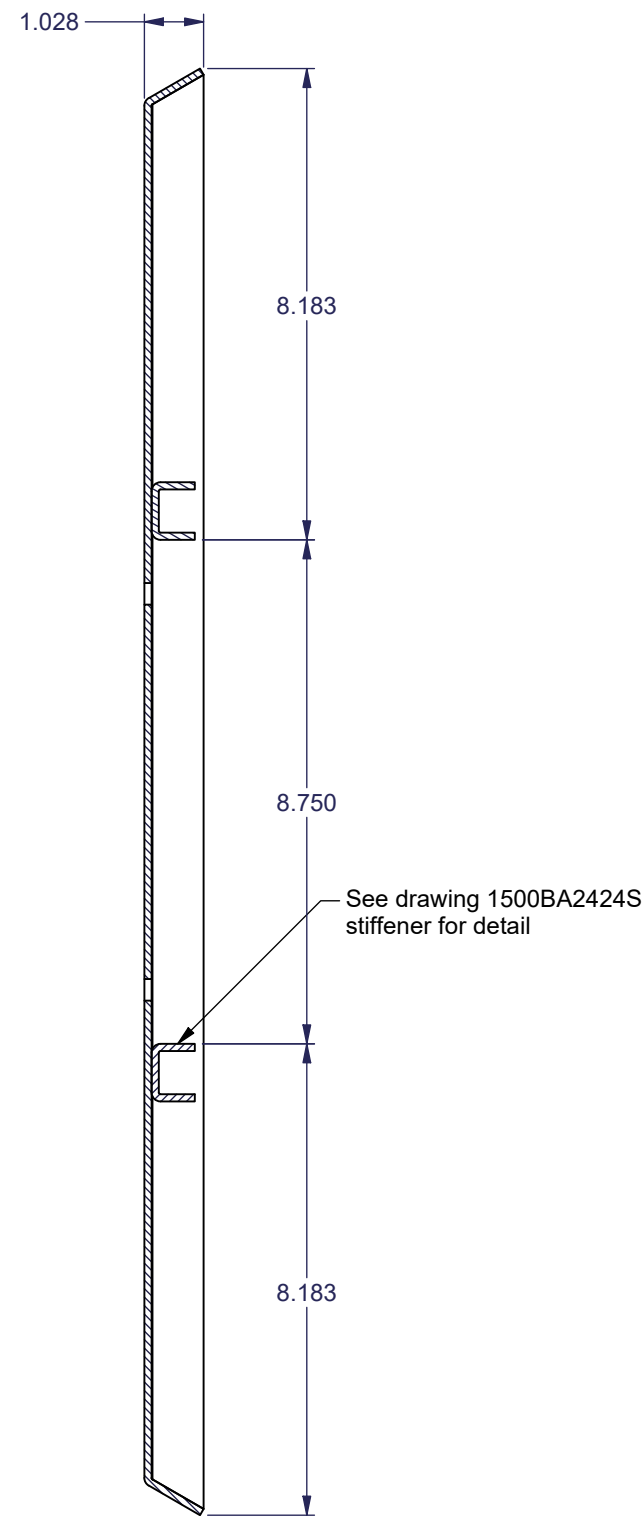
SECTION A-A
